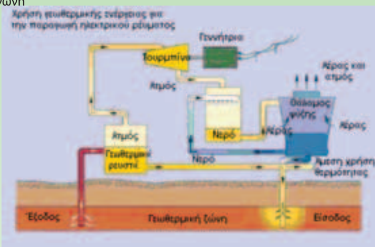
Χρήση γεωθερμικής ενέργειας για την παραγωγή ηλεκτρικού ρεύματος.
