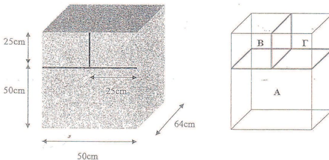
Σχήμα 2: Σύνθετη κρύπτη ραδιομολυσμένου ρουχισμού και άλλων αντικειμένων
